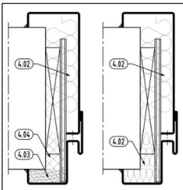
Abb. 4.6 („T 30“ / „EI2 30“)
