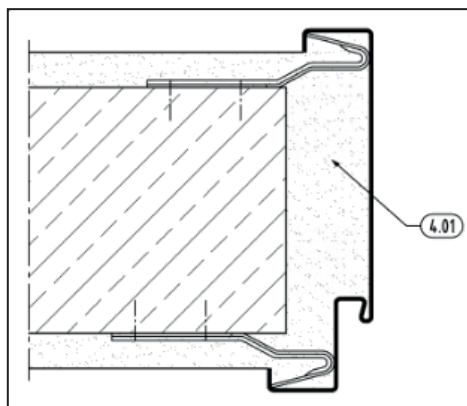
Abb. 2.4-nicht möglich bei Rauch- und Brandschutz
