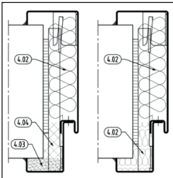
Abb. 4.2 („T 30“ / „El2 30“)
