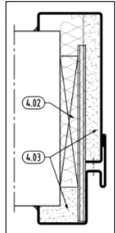
Abb. 4.7 („T90“ / „EI2 90“)
